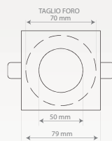
Ghiera fissa, bianco lucido / Fixed frame, glossy white
